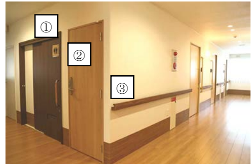
誤認識を防ぐ内装例
